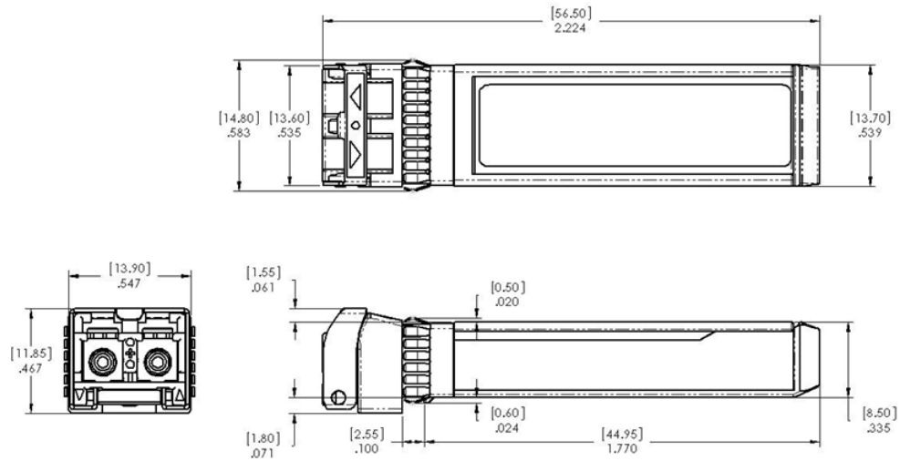
FTLF1429P3BCE
