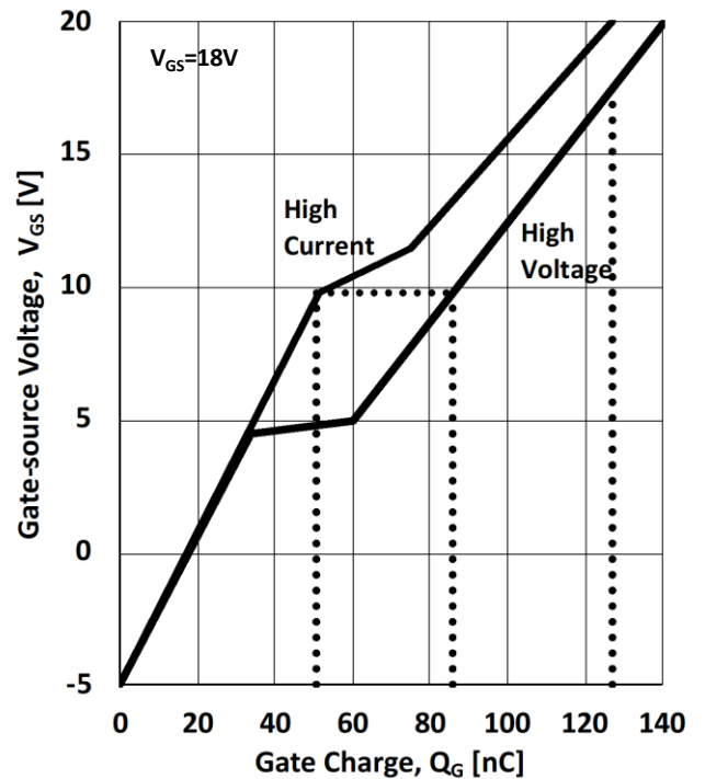
Figure 12. Gate charge V_{GS} = (-5 \dots +18 \text{ V}) ; V_{DS} = 900 \text{ V} ; I_{DS} = 30 \text{ A} ; T_J = 25^\circ C
