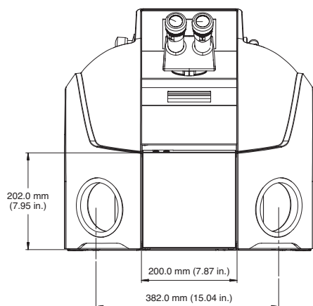
Vorderansicht
