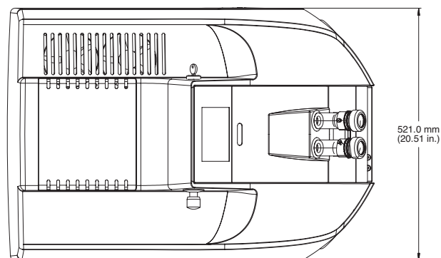
Draufsicht
